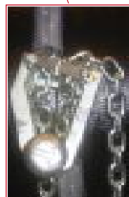
取付部拡大 調整ボルトを締め、 鎖のたるみをとる
